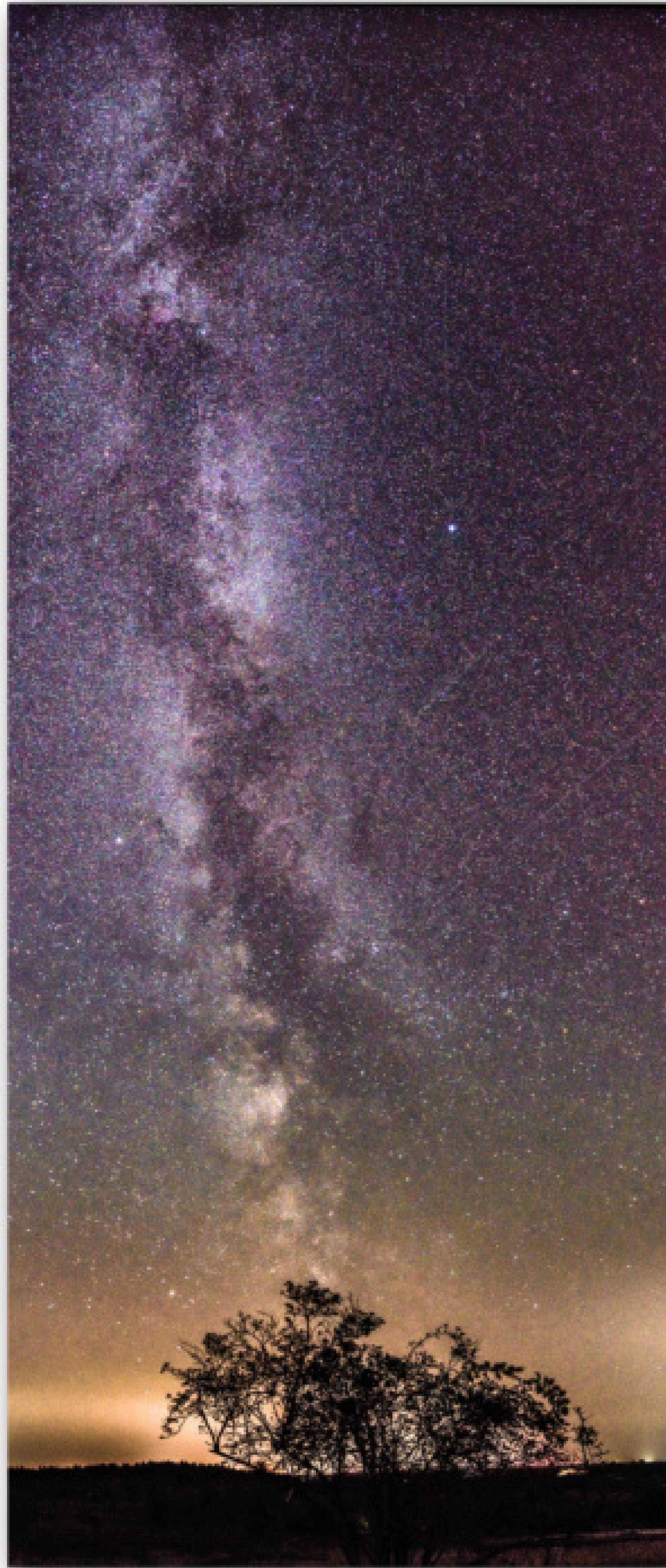
Milchstraße vom Wilseder Berg über der Lüneburger Heide + Milchstraße bei Vollmond über dem Büsenbachtal + Milchstraße über Buxtehude und der Este mit angestrahltm Kirchturm der St. Petri Kirche
