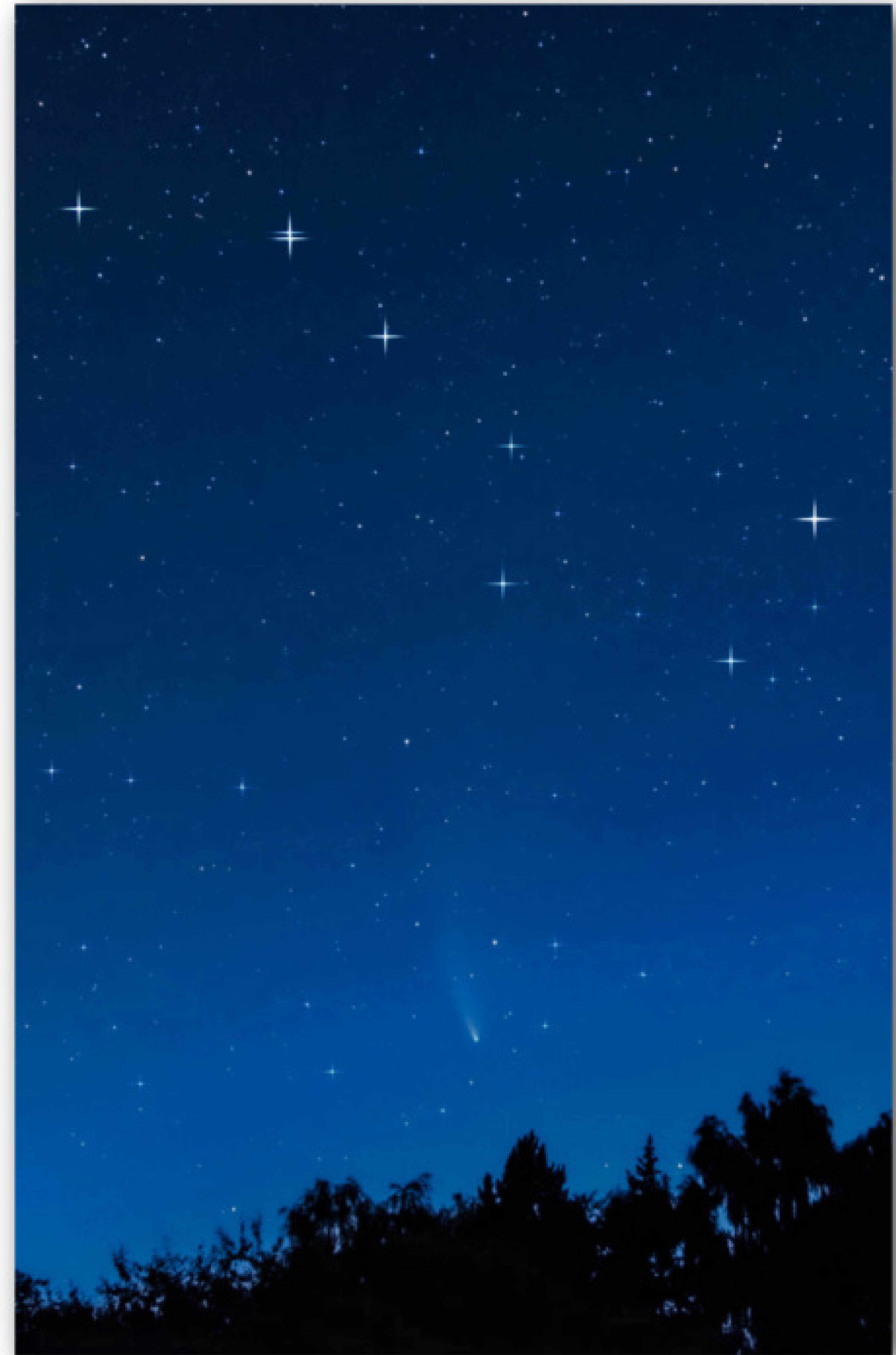
Andromeda Galaxie / M31 mit der elliptischen Galaxie M110 + Komet C/2020 F3 (Neowise) mit dem Sternbild Großer Wagen
