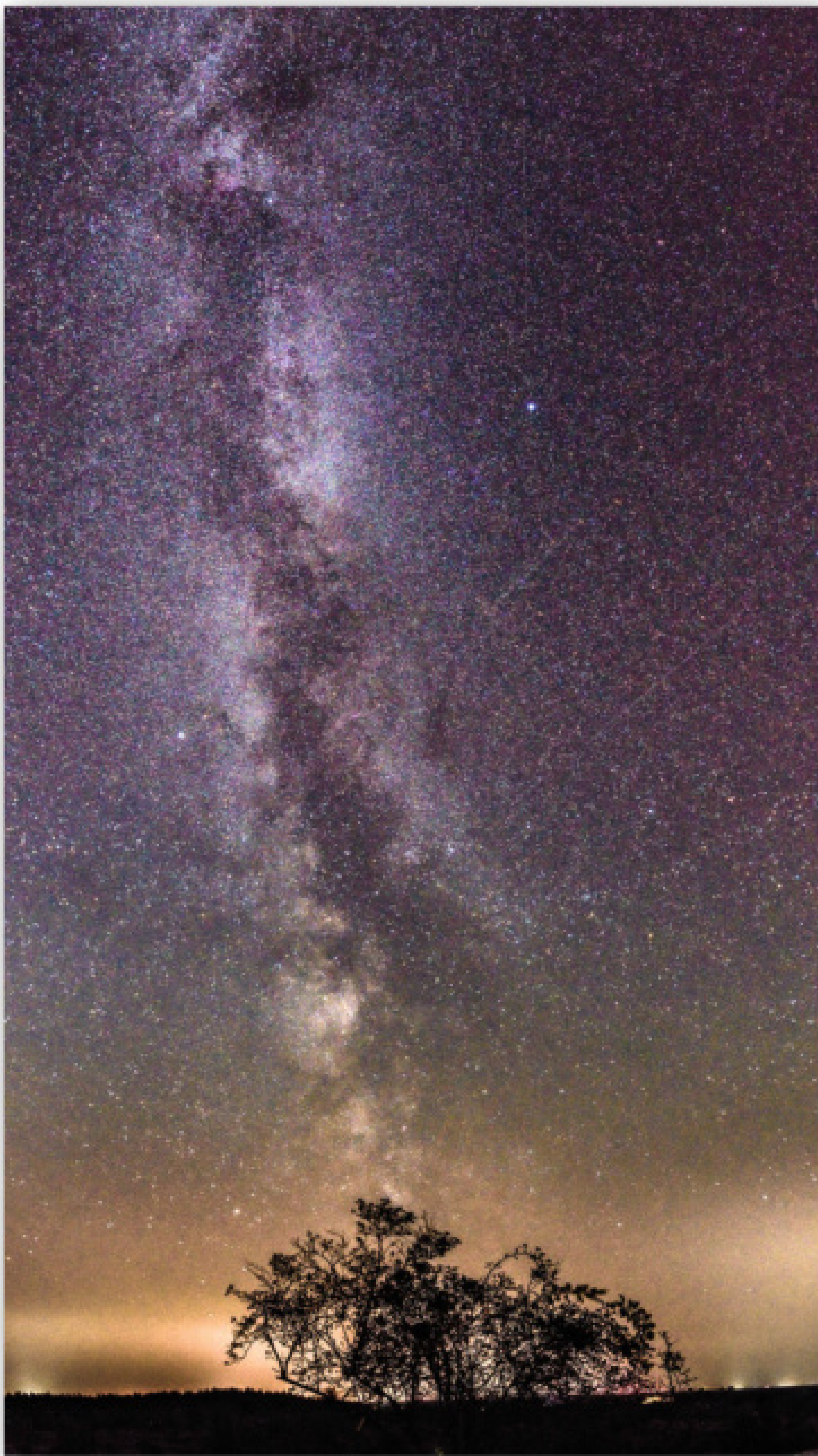
Milchstraße vom Wilseder Berg über der Lüneburger Heide + Milchstraße über Buxtehude und der Este mit angestrahlttem Kirchturm der St. Petri Kirche
